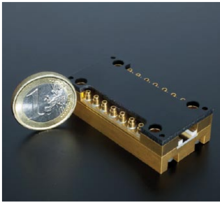
ABB. 5: Mikrosystemlichtquelle für den sichtbaren Spektralbereich. (Quelle: FBH/Schurian)
