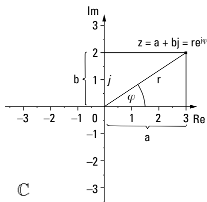
Abbildung 1.1: Polar- und Normalform einer komplexen Zahl
