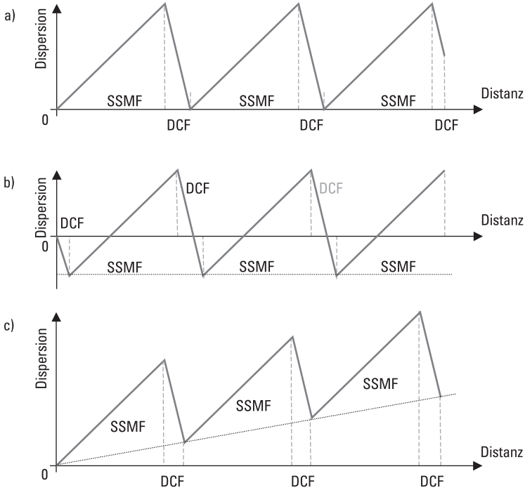
Bild 4.3 Dispersion mit Kompensation
