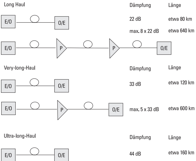
Bild 4.1 Beispiele für optische Strecken mit verschiedener Abschnittslänge
