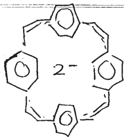
A 26 \pi -perimeter
